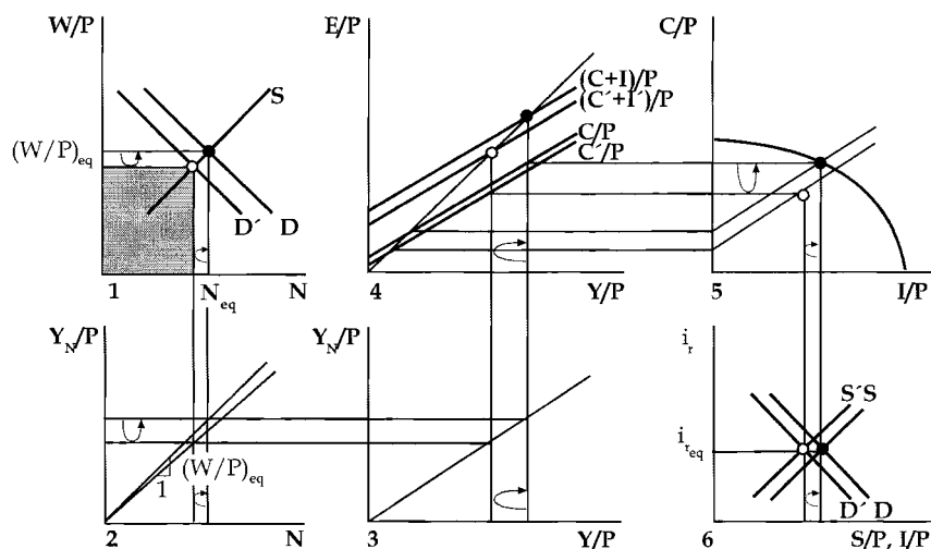
Figura 11.2. Desequilibrio monetario (en la estructura basada en el trabajo).
